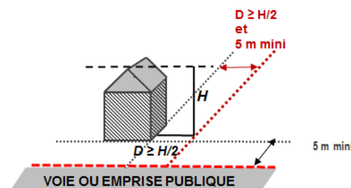
Schéma illustratif : implantations en limites séparatives en zones UBs et UBepa et pour les équipements d'intérêt collectif et services publics
