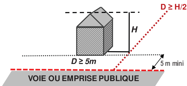
Schéma illustratif : implantations en limites séparatives en zone AUc
